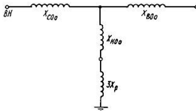
Рис. 2. Нетрадиционная схема замещения нулевой последовательности автотрансформаторов с реактором в нейтрали
