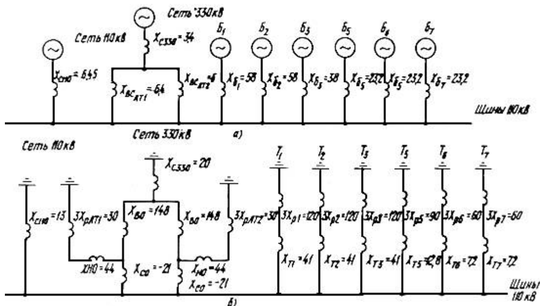
Рис. 4. Схемы замещения сети 110 кВ ГРЭС-1:
