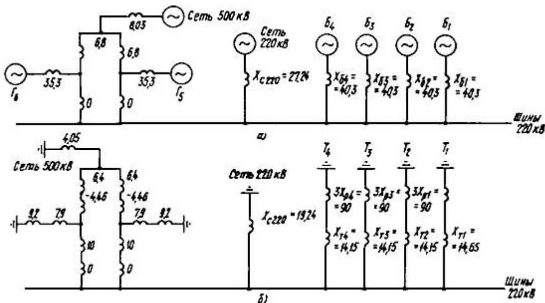
Рис. 5. Схемы замещения сети 220 кВ ГРЭС-2:
