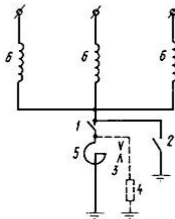
Рис. 1. Схема включения реакторов в нейтрали трансформаторов и автотрансформаторов:
